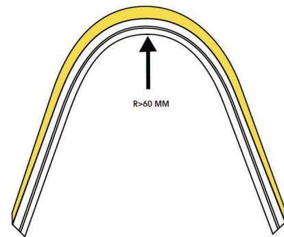
TOP VIEW - FLESSIONE VERTICALE R<60 mm
