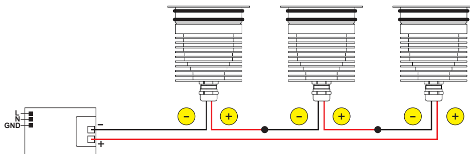
Schema di connessione in serie per versione 350 / 500 / 700mA Connection diagram for 350 / 500 / 700mA version
