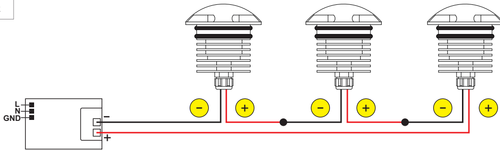
Schema di connessione in serie per versione 350mA Connection diagram for 350mA version
