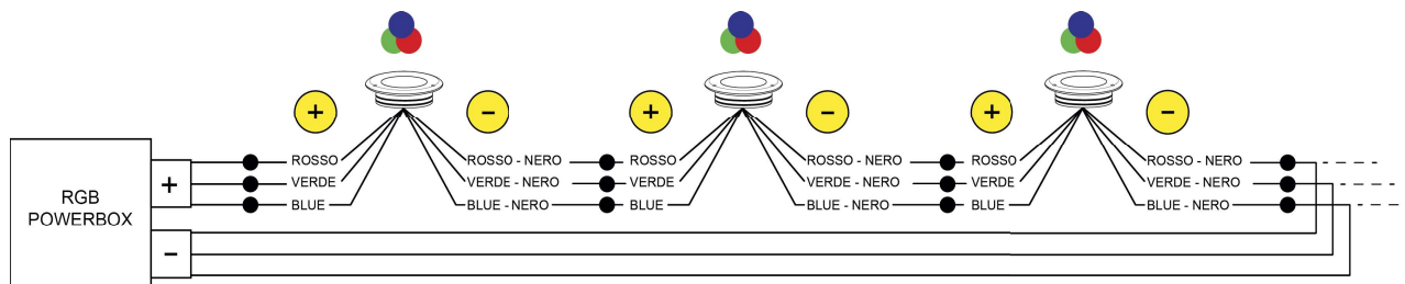
Schema di connessione per versione RGB
